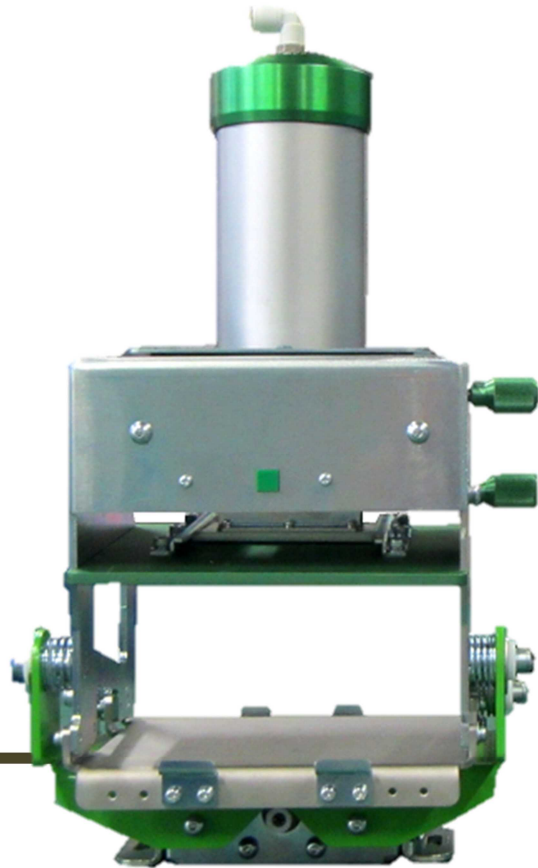
■ マルチクランプ(オプション) 通常～大型のゴム型まで対応可能なマルチクランプが装着可能です。 クランプ位置の X 軸 Y 軸が調整可能です。
